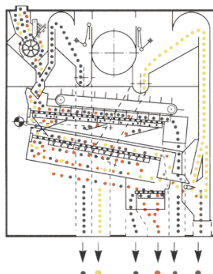
Sitový systém, 2-sitový
