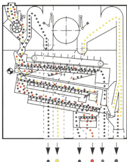
Sitový systém, 3-sitový
